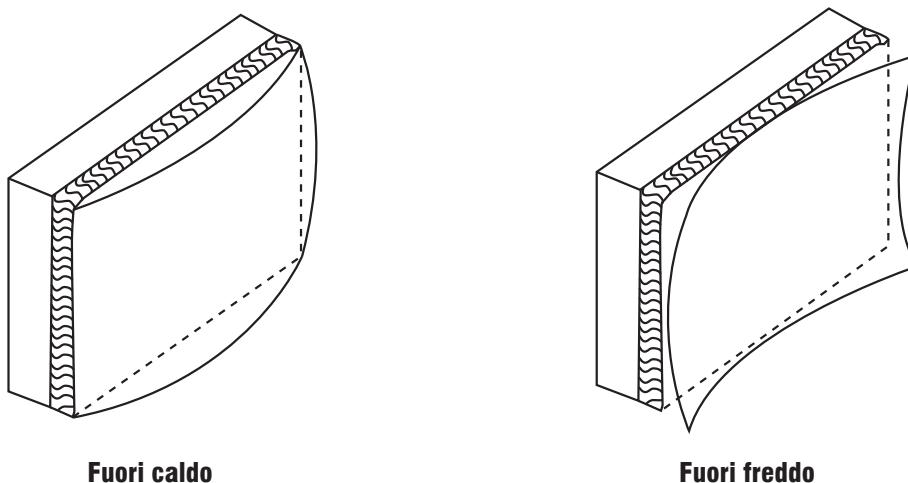
FIGURA 4: l'applicazione del collante può avvenire con il metodo di incollaggio a cordolo perimetrale e punti centrali (figura 5) o a tutta superficie (figura 6)
