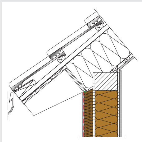
FIGURA 38: collegamento a copertura inclinata
