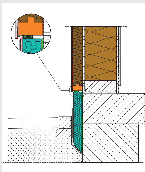
FIGURA 36: zoccolatura
