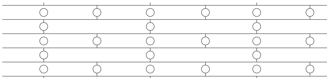
FIGURA 15: tassellatura con pannelli MW a fibre verticali
