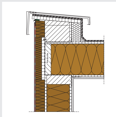
FIGURA 39: collegamento a copertura piana
