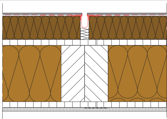
FIGURA 37: giunto di dilatazione verticale
